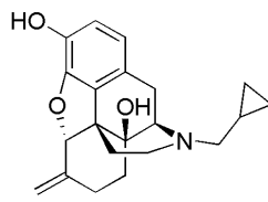
Nalmefene
