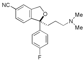
Escitalopram
