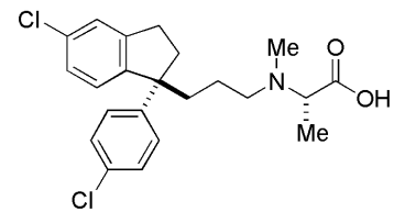
Lu AA26778
