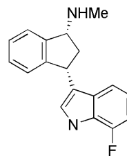
Lu AA42202
